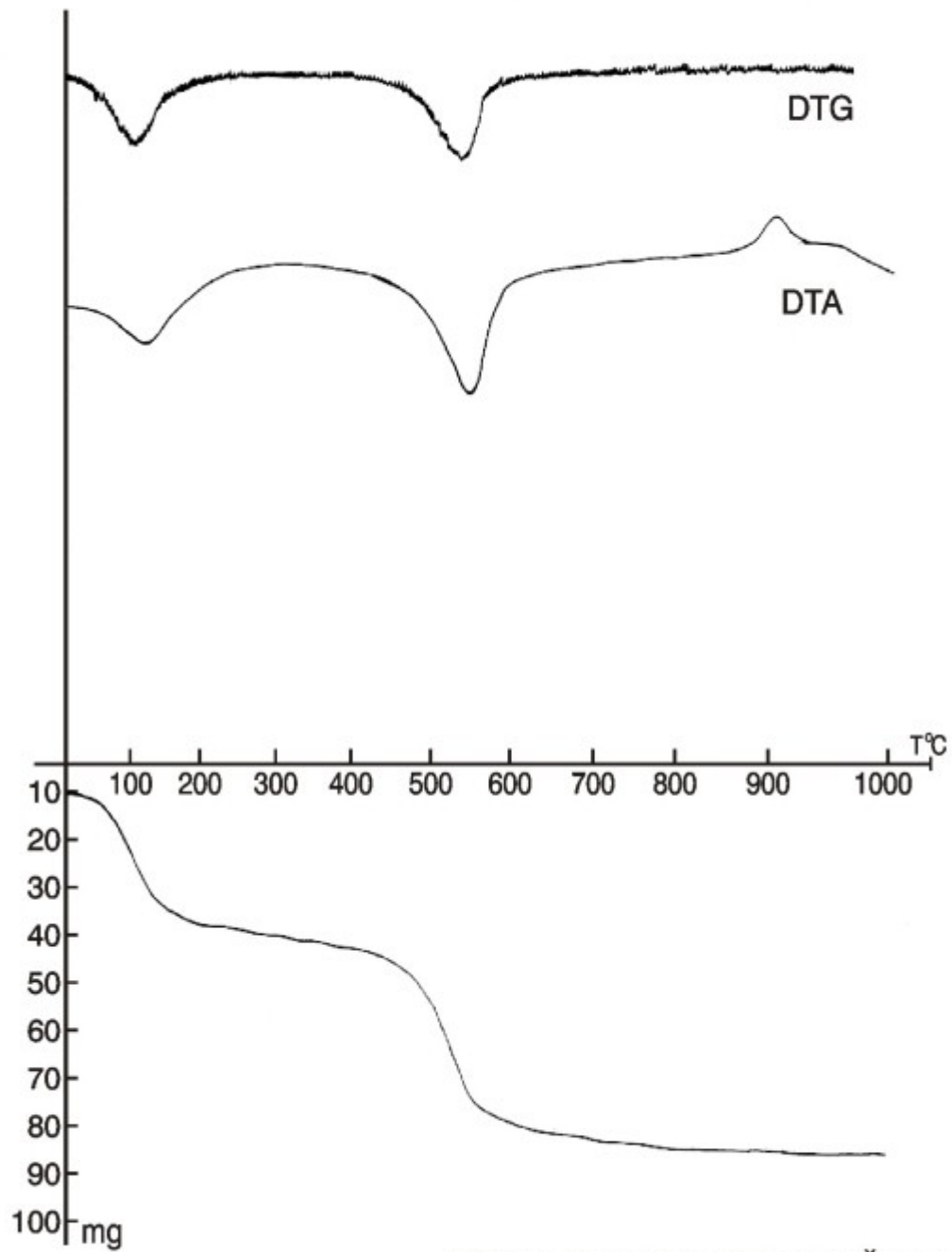
DIFERENCIJALNO TERMIČKA I TERMO GRAVIMETRIJSKA ANALIZA GLINA KOŠARNO
